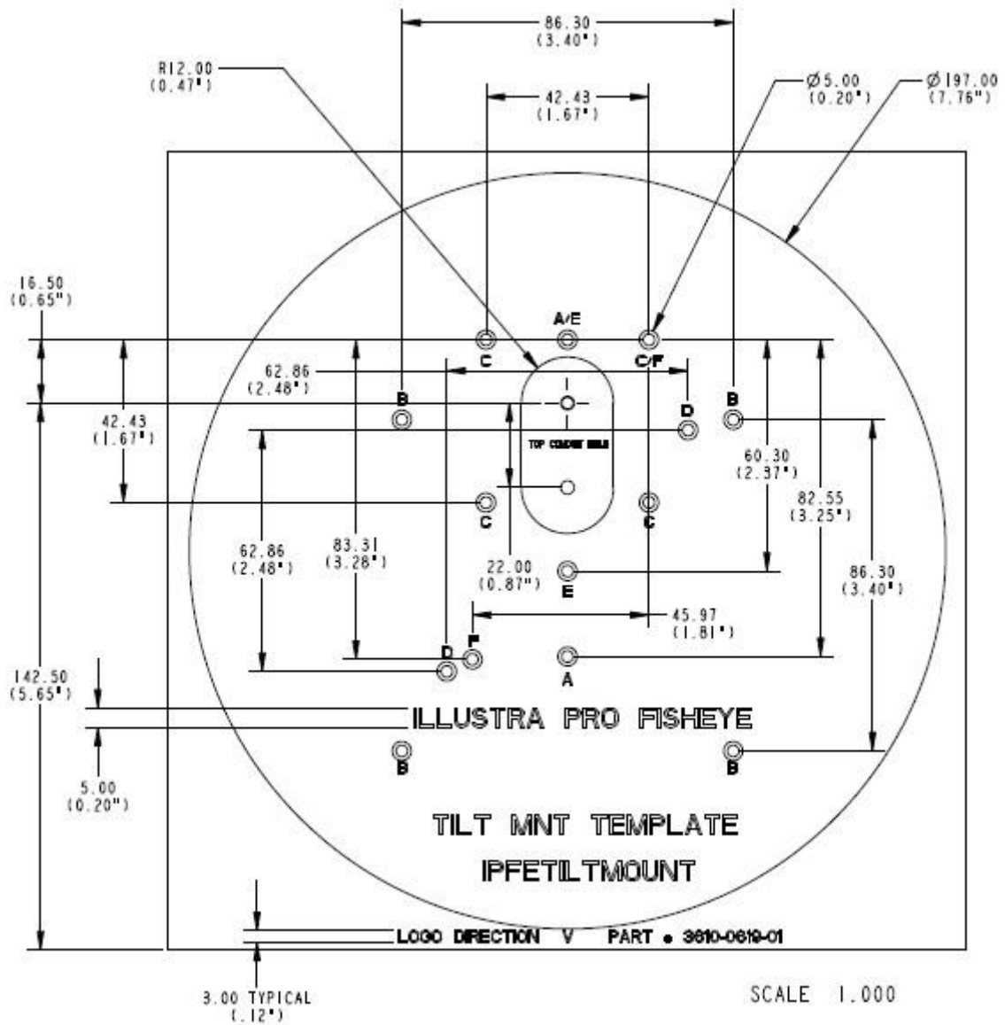
Figure 9 Gabarit pour support incliné
