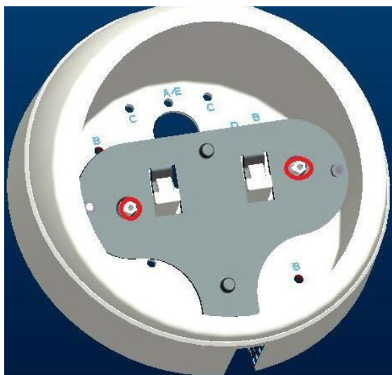
Figure 7. Ensemble base de caméra avec support incliné installé
